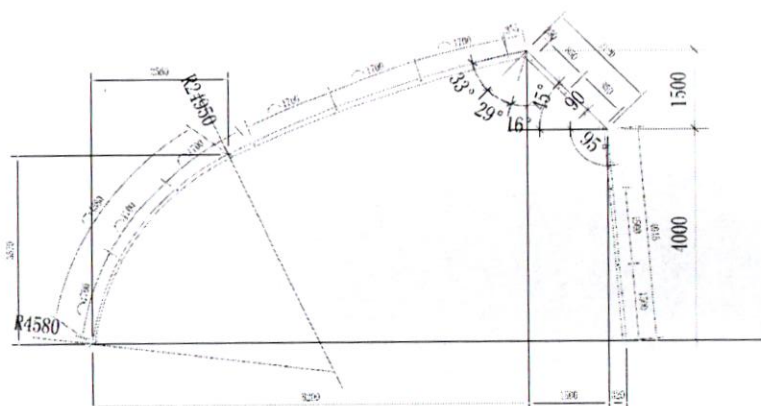
图 2 全落地式日光温室钢结构骨架示意图（无后墙温室）
